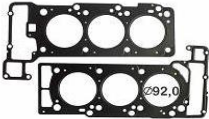
25202 MLS - 0,65 MM - CIL. 92 MM JUNTA CABEÇOTE - PAR
